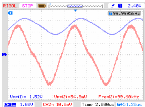
Grafico 7 – Señal acondicionada 100kHz
