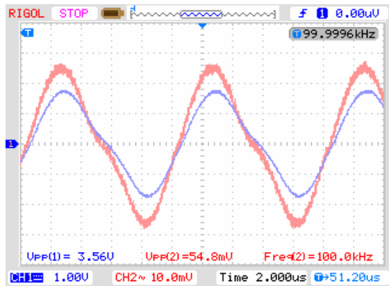
Grafico 6 – Señal sin acondicionar 100kHz
