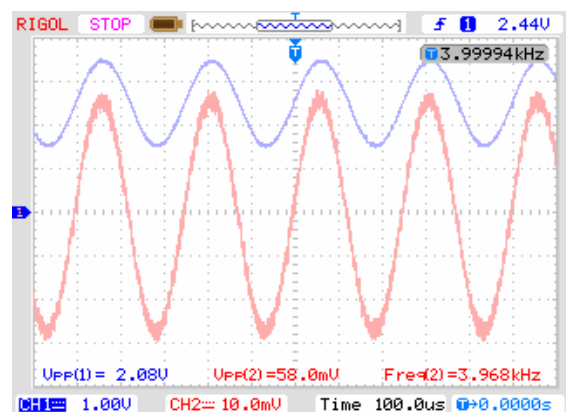
Gráfico 5 – Señal acondicionada 4kHz
