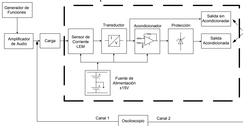
Fig. 1 – Esquema de conexionado para el ensayo
