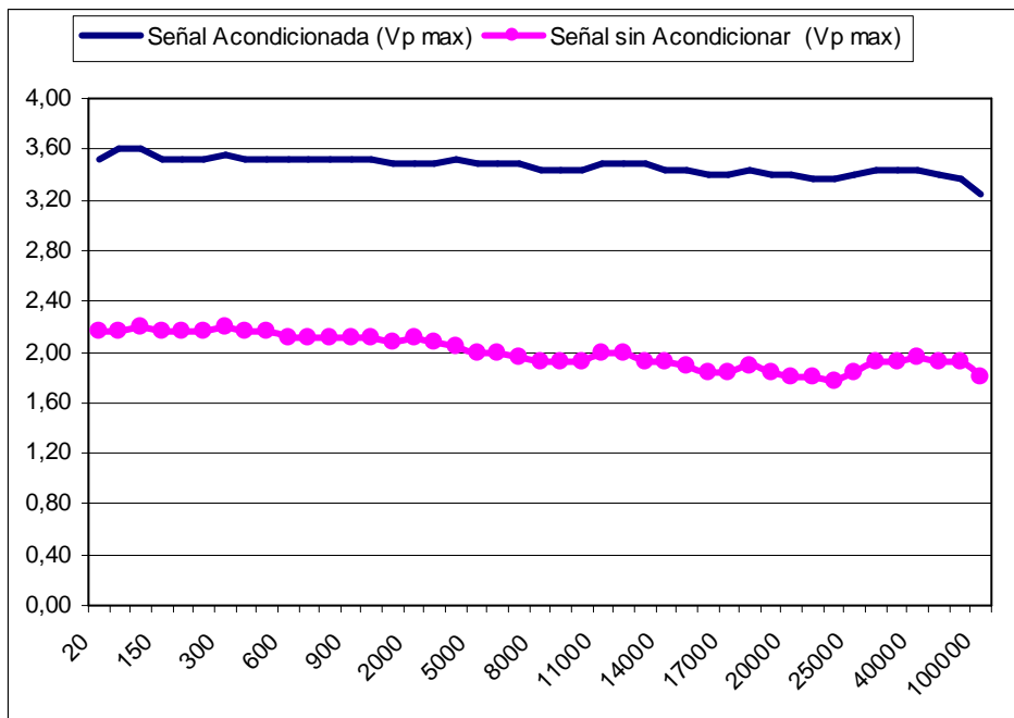
Gráfico 2 – Respuesta de la salida acondicionada y sin acondicionar en función de la frecuencia
