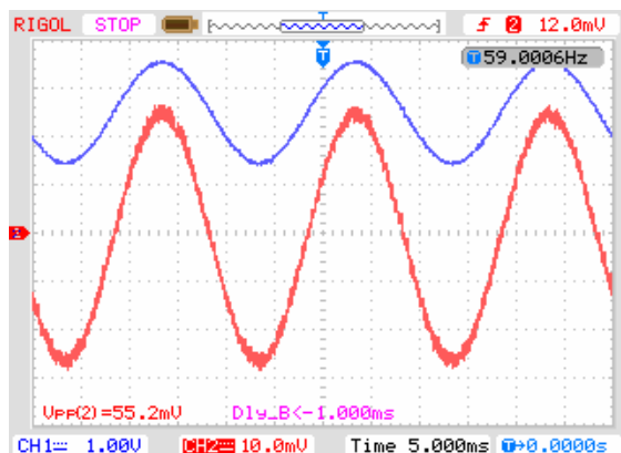
Gráfico 3 – Señal acondicionada 60Hz
