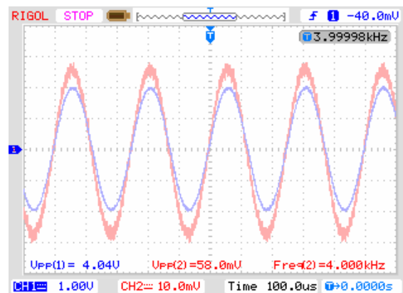
Gráfico 4 – Señal sin acondicionar 4kHz
