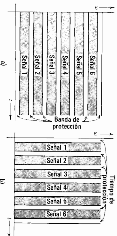
Figura 5.15 Representación en un espacio de comunicación de la multicanalización por división de frecuencia y de tiempo.
