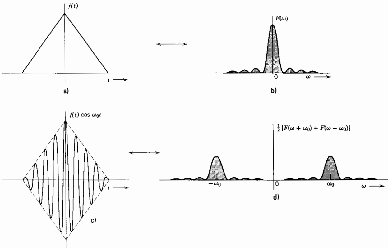
Figura 1.39 Efecto de la modulación en el espectro de frecuencias.
