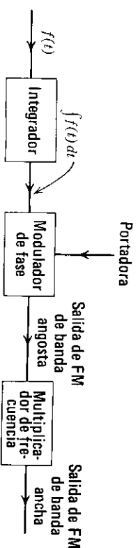
Figura 4.8 Representación en bloques de la generación indirecta de FM.
