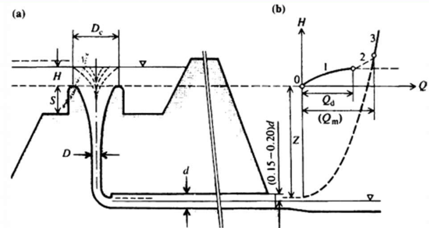
Figura 4.13 Vertedero de pozo.
