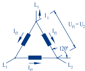
Figura 1.7a - Ligações
