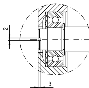
DETALHE X SOMENTE P/ FORMA J
