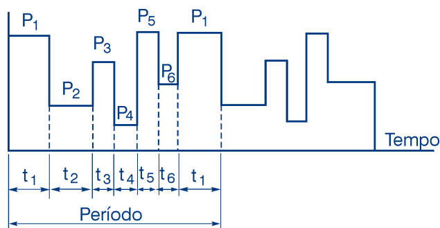
Figura 5.18 - Funcionamento contínuo com solicitações intermitentes
