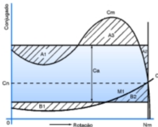
Figura 3.5 - Determinação gráfica do conjugado médio de aceleração
