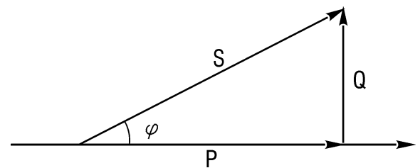
Figura 1.2 - Triângulo de potências (carga indutiva)
