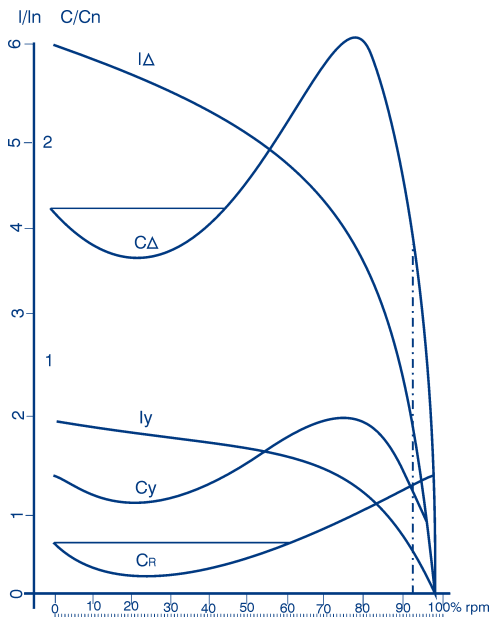
Figura 2.11 I_{\Delta} - corrente em triângulo I_Y - corrente em estrela C_{\Delta} - conjugado em triângulo C_Y - conjugado em estrela C/C_n - relação entre o conjugado do motor e o conjugado nominal I/I_n - relação entre a corrente de partida e a corrente nominal C_r - conjugado resistente
