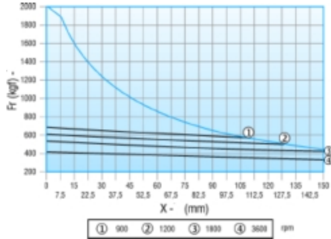
Carcaça 200
