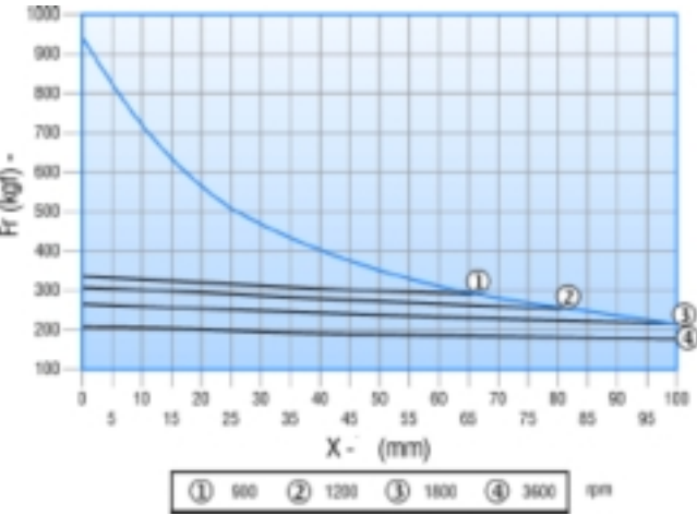
Carcaça 132
