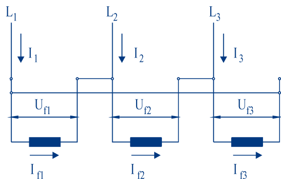
Figura 1.7a - Ligações
