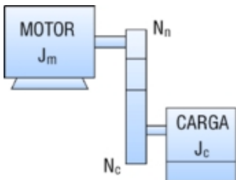
Figura 3.3 - Momento de inércia em rotações diferentes
