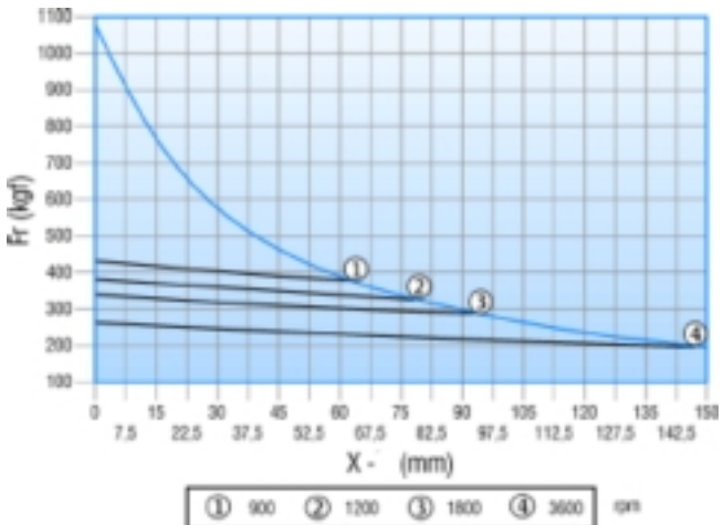
Carcaça 160
