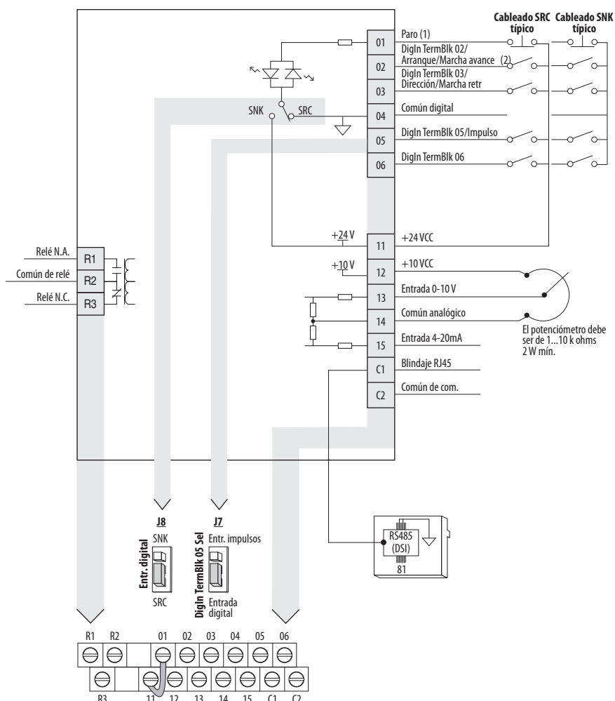
Diagrama de bloques del cableado de E/S de control del PowerFlex 523
