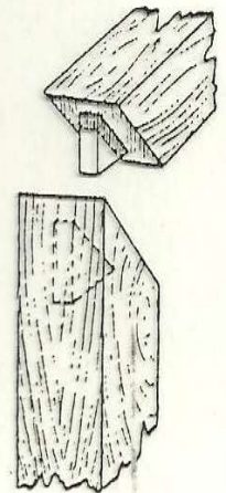
INGLETE A CAJA Y ESPIGA
