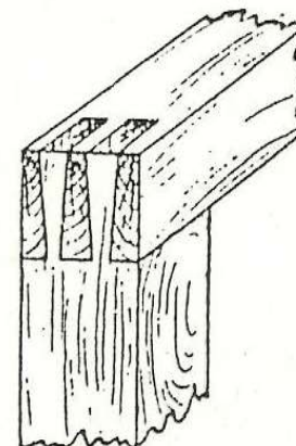
A DOBLE COLA DE MILANO
