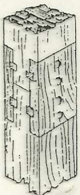
A TOPE CON PLATABANDAS REBAJADAS
