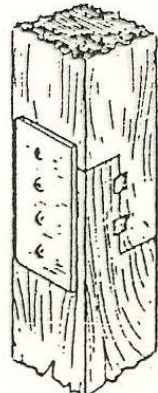
A MEDIA MADERA CON CUBRE-JUNTA METALICA Y CUÑAS
