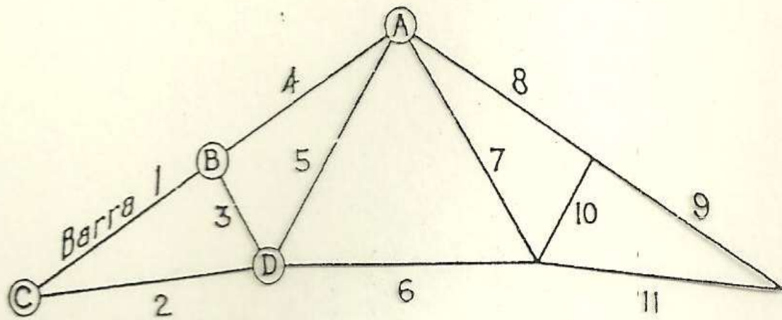
ESQUEMA DE UNA CERCHA O CABRIADA
