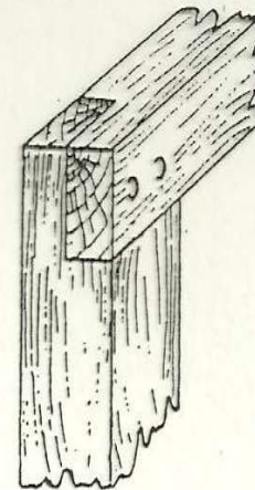
A MEDIA MADERA
