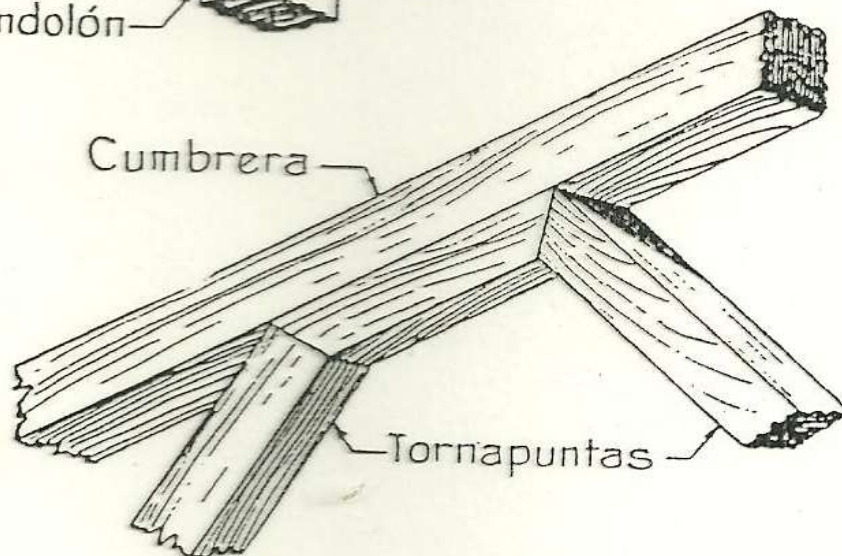
NUDO DE UNA ARMADURA CON SUPLEMENTO
