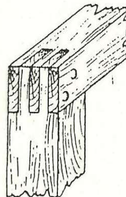
A DOBLE HORQUILLA
