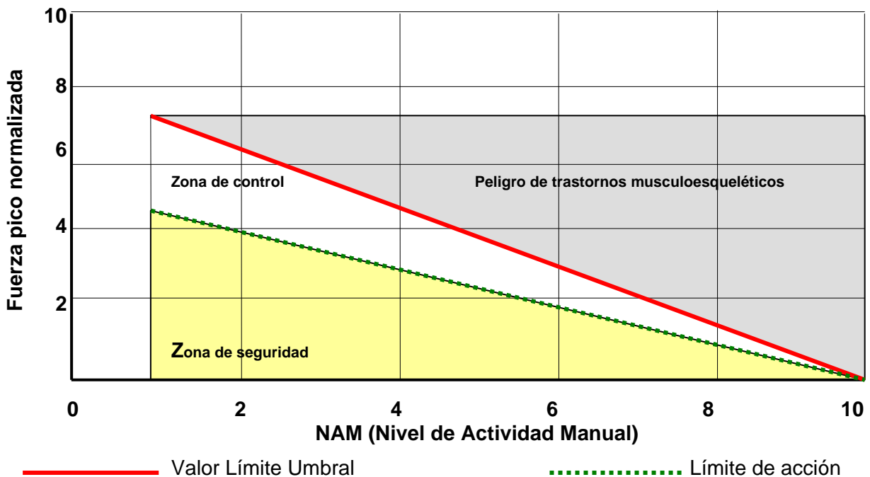
Figura 1. El valor para reducir los trastornos musculoesqueléticos relacionados con el trabajo en la “actividad manual” (AM) y la fuerza máxima (pico) de la mano. La línea continua representa el valor límite umbral. La línea de puntos es un límite de Acción para el que se recomienda establecer controles generales.
