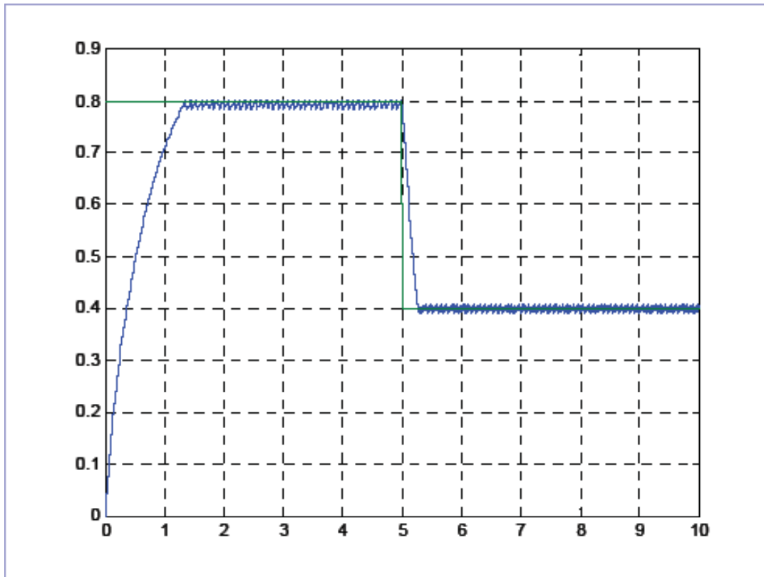
CONTROL ON-OFF CON HISTÉRESIS = 0
