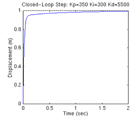
ACCIÓN “P+I+D”
