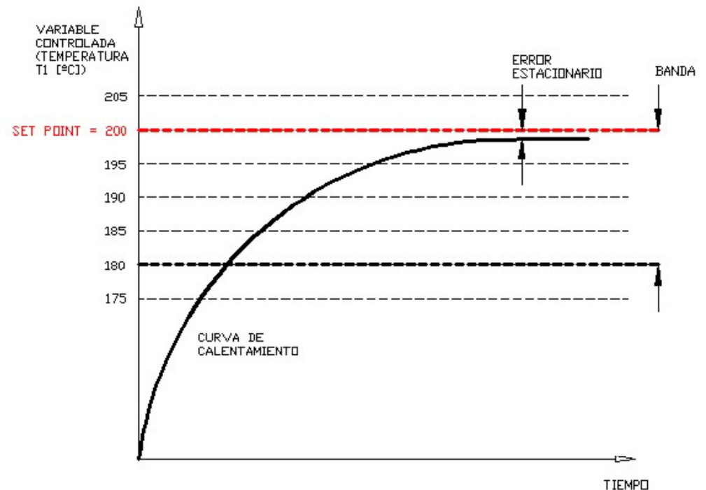
CARACTERÍSTICA DINÁMICA DEL HORNO DE CALENTAMIENTO DIRECTO CON CONTROL PROPORCIONAL
