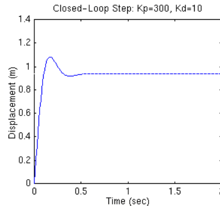
ACCIÓN “P+D”
