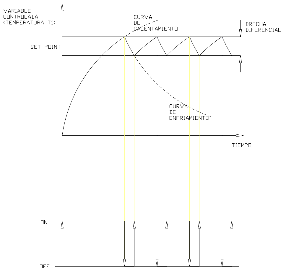
DIAGRAMA DE MANIOBRAS DEL CONTACTOR
