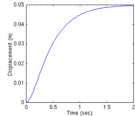
ACCIÓN “P+I+D”
