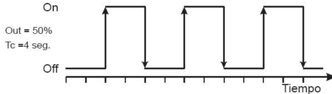
Salida Modulada PWM
