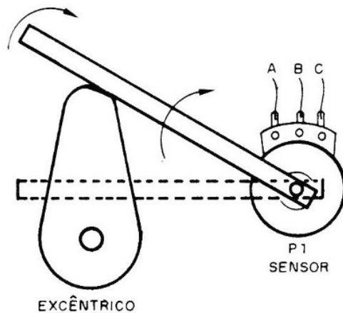
Figura 1 – Accionamiento para un sistema excéntrico
