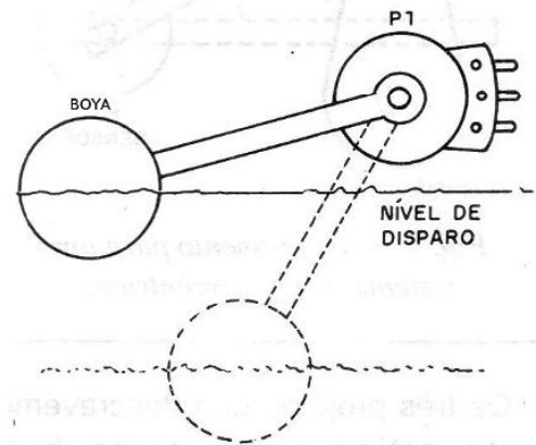
Figura 10 – usando el sensor en una caja de agua
