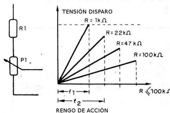
Figura 12 – Cambiando la pista de actuación con una resistencia
