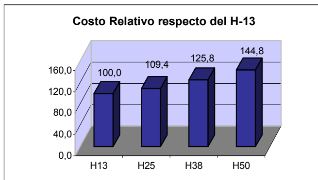
Figura 1: Costo relativo de distintas clases de hormigón tomando como valor de referencia (100) al H-13. Se supone que en todos se emplea la misma categoría de cemento y el mismo conjunto de agregados.
