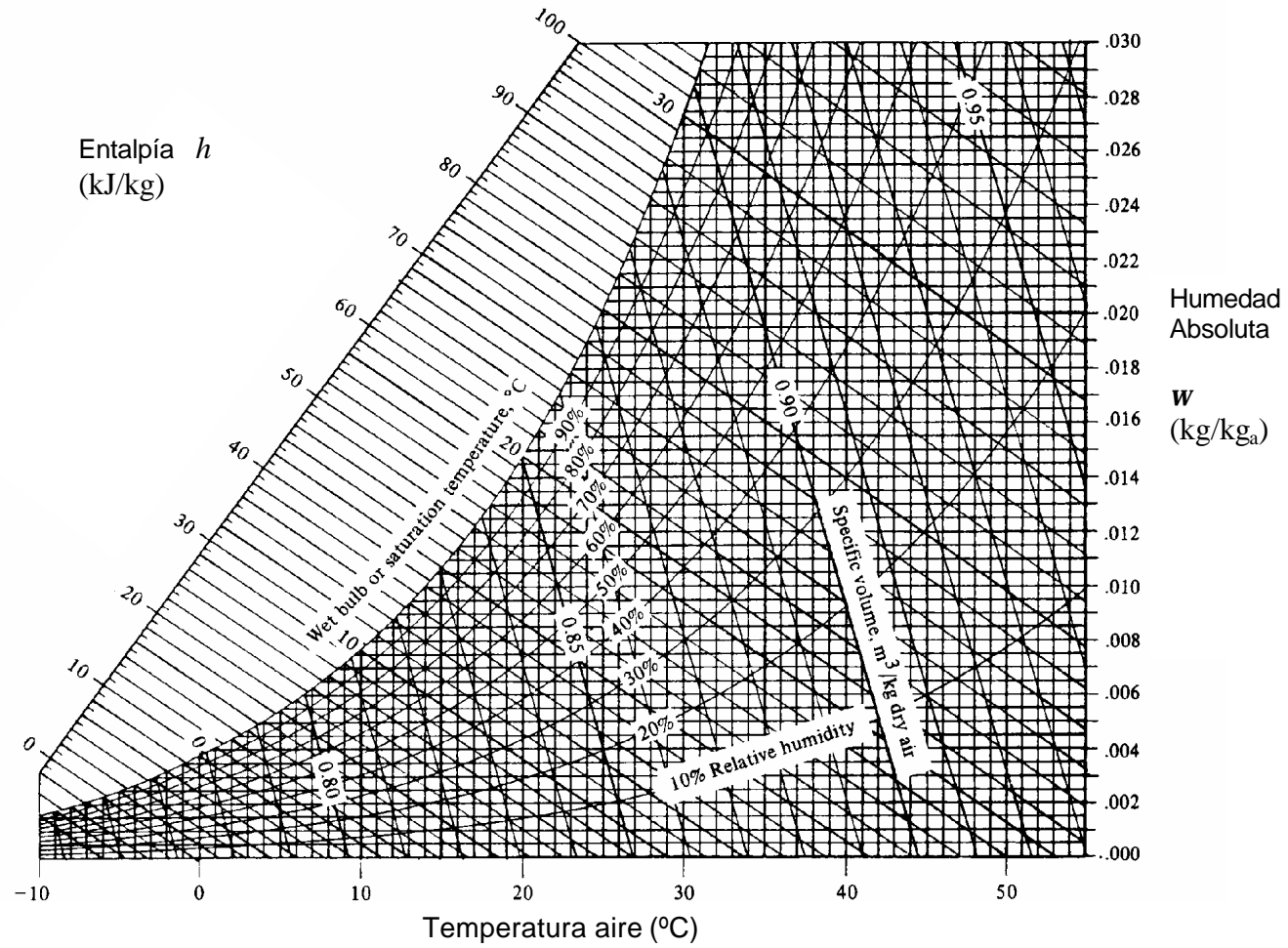
6. TABLA: Carta Psicrométrica (ASHRAE)
