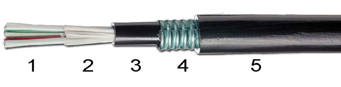
Figura 2: Cable de fibra óptica de estructura holgada (DPESP de OPTRAL) 1. Tubos plásticos conteniendo fibras a 250 \mu\text{m} 2. Elemento resistente periférico (Hilaturas de fibra de vidrio) 3. Cubierta interior PE 4. Armadura de chapa de acero corrugado 5. Cubierta exterior PE
